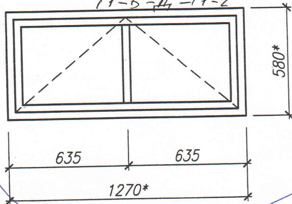
Схема оконного блока ОК-3
