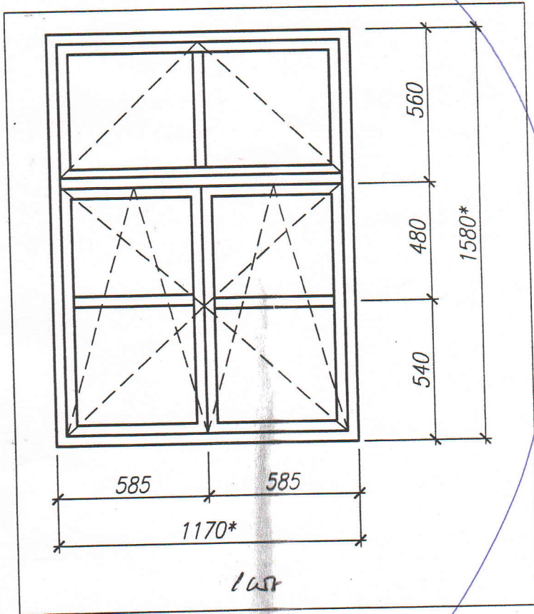
Схема оконного блока ОК-1* ОД 10 1580 x 1170 П/О СП 2 Ч О Г
